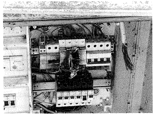
Q.E. pubblica illuminazione Rendola
